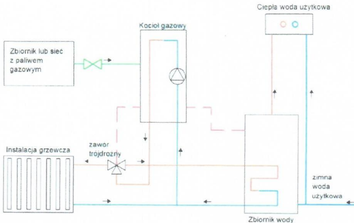
Rys. 2 — Schemat ideowy instalacji ciepłej z kotłem gazowym
