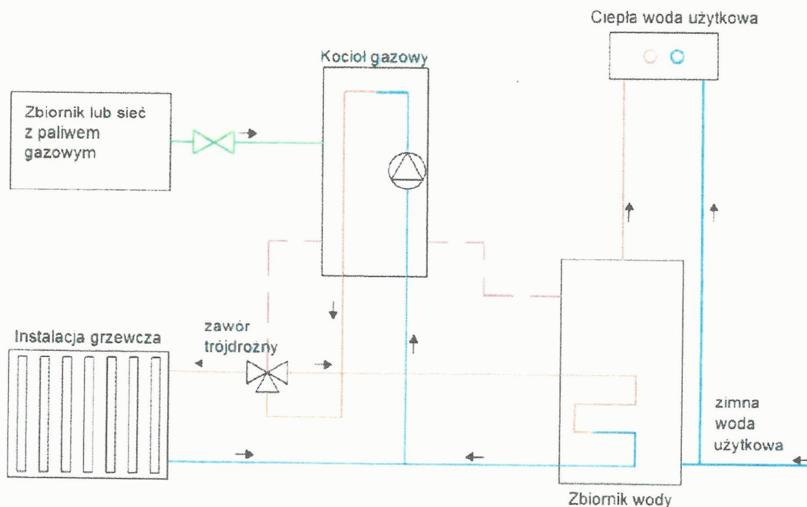
Rys. 2 — Schemat ideowy instalacji cieplnej z kotłem gazowym
